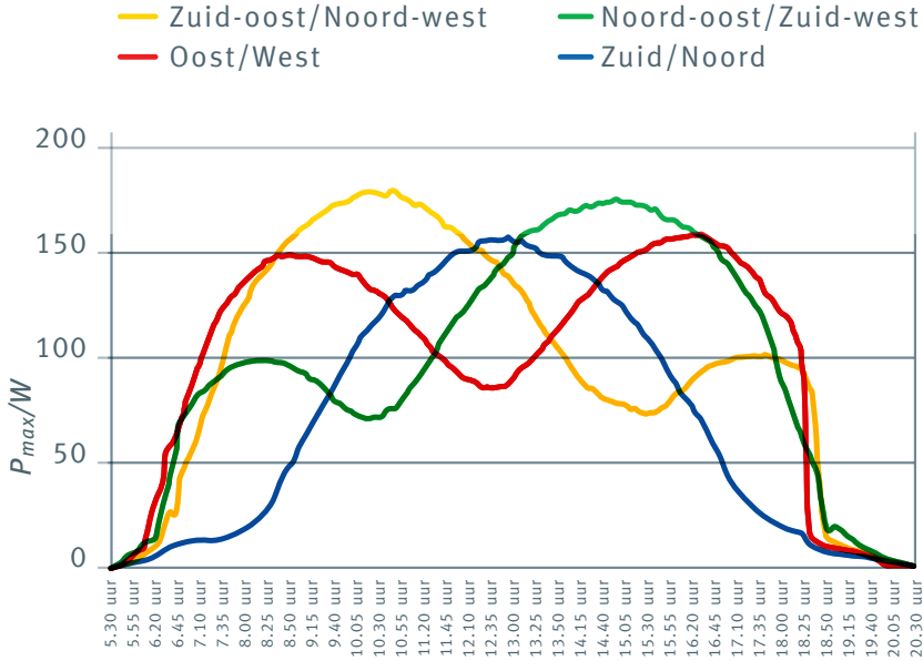
Maximale prestaties van OPTIGRÜN SOLAR SOLon in verschillende oriëntaties gedurende de dag
